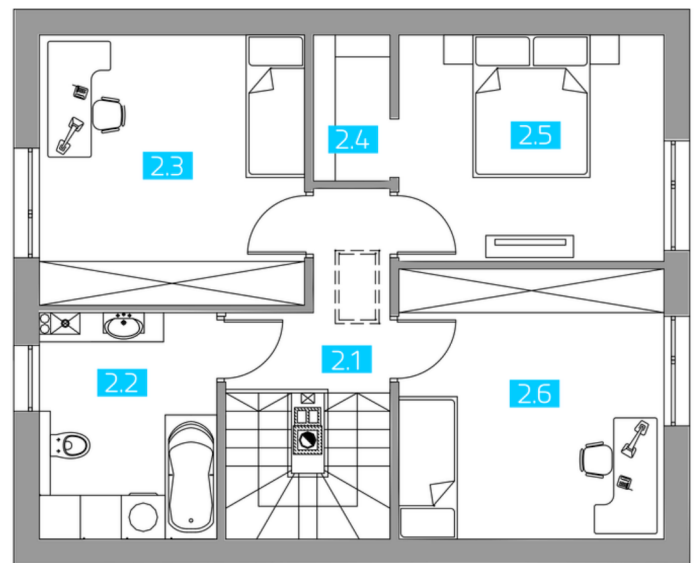
RZUT PODDASZA
