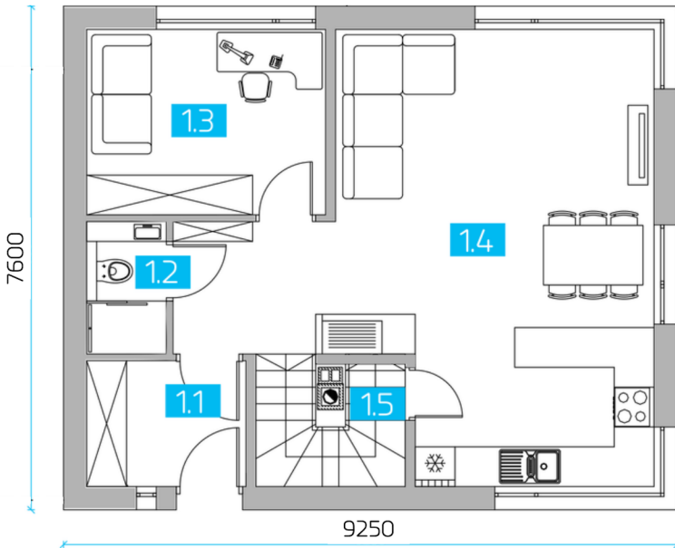
RZUT PARTERU
