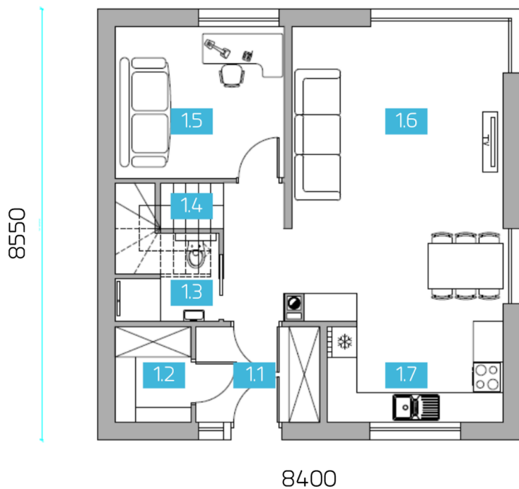
RZUT PARTERU
