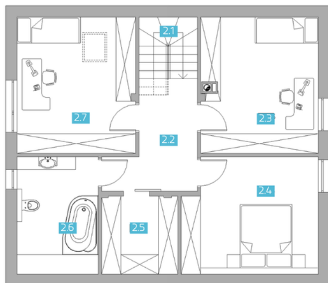
RZUT PODDASZA
