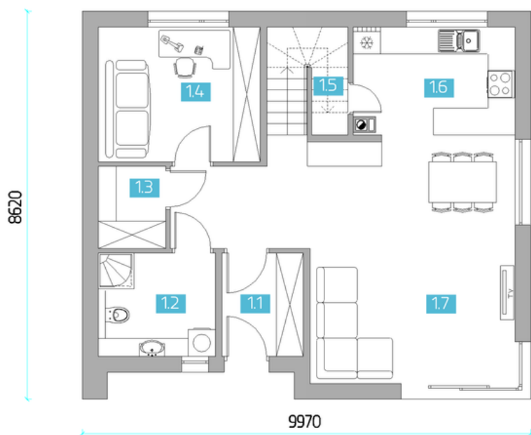
RZUT PARTERU
