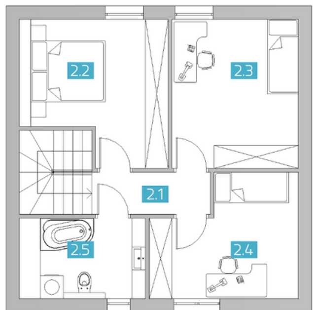
RZUT PODDASZA
