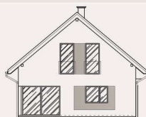
ELEWACJA TYLNA
