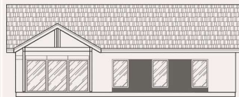
ELEWACJA TYLNA
