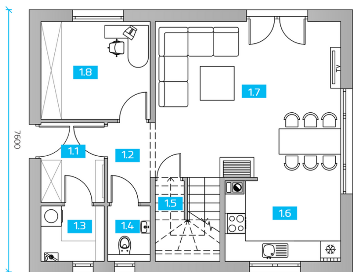
RZUT PARTERU
