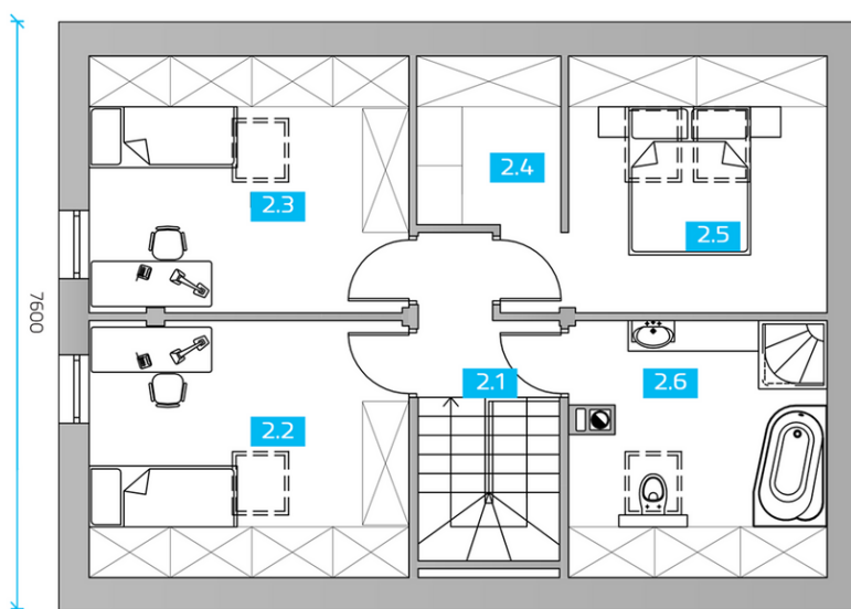
RZUT PODDASZA
